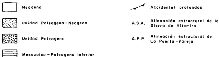
Fig. 2.1 - Esquema tectónico simplificado de la Hoja de Auñón
