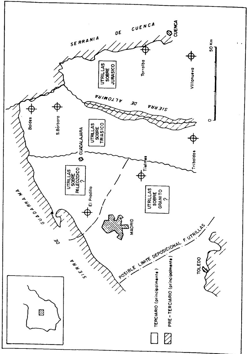
Fig. 2.7 - Sustrato de la Fm. Utrillas en el ámbito de la Cuenca del Tago. Depresión Intermedia. (Según RACERO, 1988)
