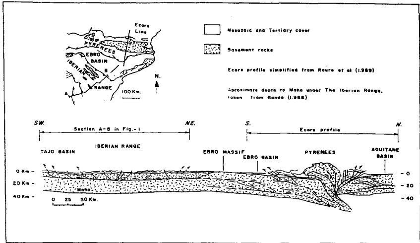
Fig. 2.13 - Sección crustal del sistema compressivo Pirineos-Cordillera Ibérica, según HERNALZ et al (inédito).
