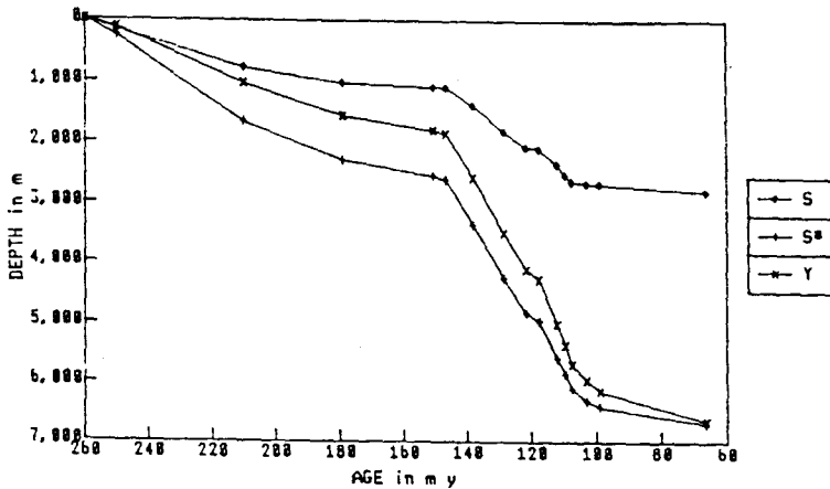
Fig. 4.4 - Curvas de subsidencia en el depocentro de la Cuenca del Maestrazgo. Se considera el efecto de compactación diagenética de los sedimentos. S*, subsidencia total; Y, subsidencia observada; S, subsidencia tectónica (según SALAS y CASAS, 1990).
