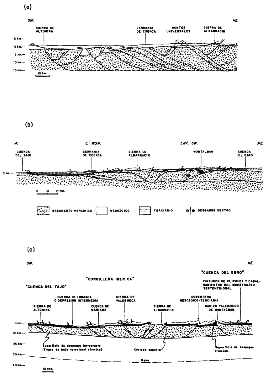
Fig. 2.12 - Cortes geológicos profundos de la Cordillera Ibérica mostrando la imbricación del basamento por encima de una superficie de despegue intracrustal, (a) según VIALLARD, 1989; (b) según GUIMERA y ALVARO, 1990; (c) según HERNÁIZ et al (inédito).
